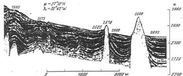
Рисунок 21. Алжирская котловина. Купола, прорывающие толщу осадков. Слева купола не прорвали толщу, но над ними в осадках складки нагнетания [Живаго 1994]
