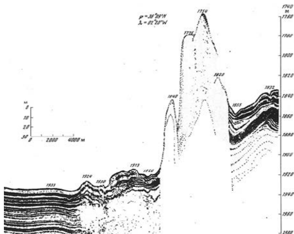
Рисунок 20. Восточно-Альборанская котловина Средиземного моря. Сквозное протыкание осадочной толщи соляными куполами. Справа скала глубин. Поверхность осадков находится на глубине 1920 и 1855 м, а вершины куполов — 1840–1754 м [Живаго 1994]
