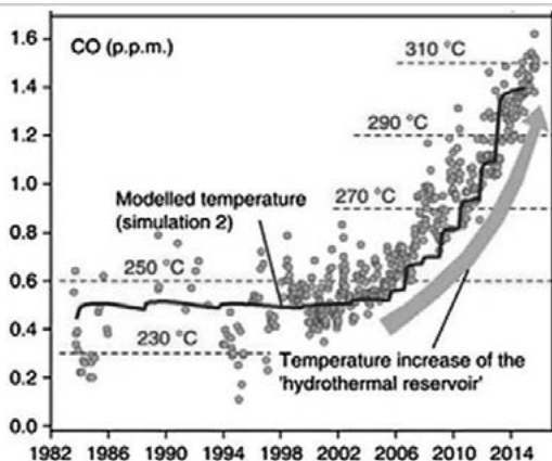
Рисунок 60. Изменение температуры в гидротермальном резервуаре Флегрейских полей с 1982 по 2014 год по данным Р. Морети с соавторами [Флегрейские поля 2018]
