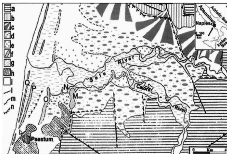
Рисунок 74. Геологическая схема грабена залива Солерно, где располагается Пестум:
